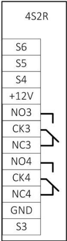
Рис.1. Схема подключения.
