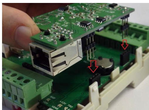
Рисунок 1. Установка концентратора СЕМ
