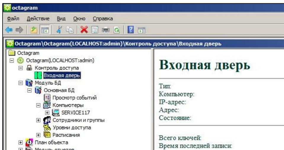
Рисунок 8 – Переименованный контроллер
