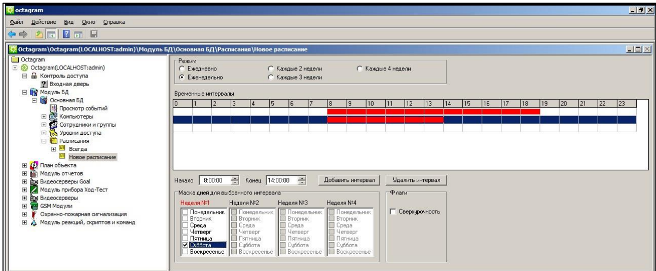
Рисунок 17 – Настройка расписания
