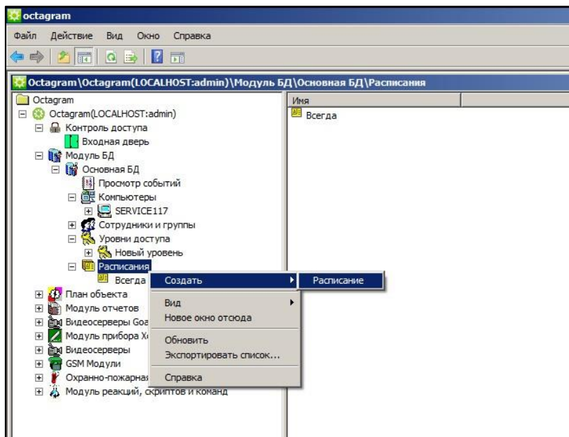
Рисунок 13 – Создание расписания
