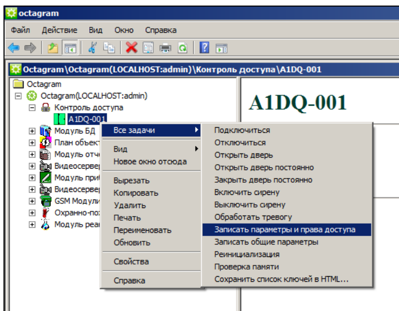
Рисунок 24 – Запись параметров
