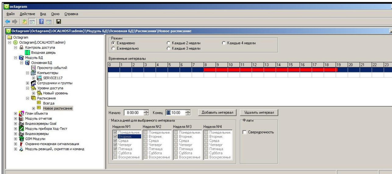
Рисунок 14 – Добавление интервала
