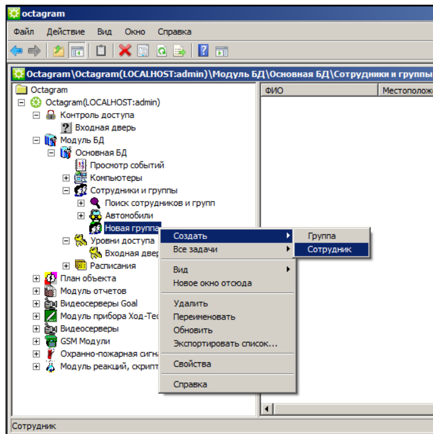
Рисунок 21 – Создание сотрудника
