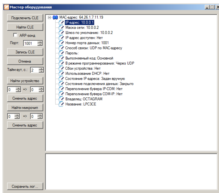
Рисунок 3 Настройка концентратора
