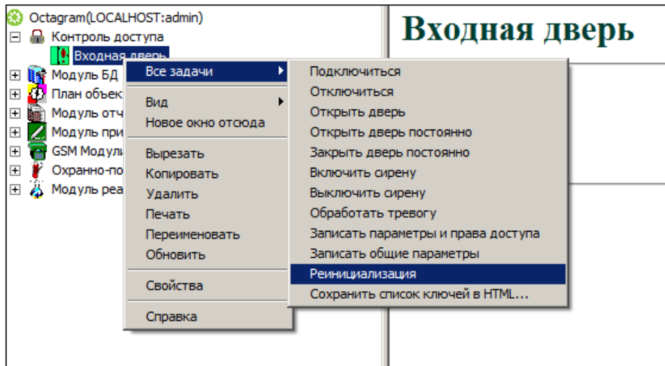
Рисунок 9 – Реинициализация контроллера
