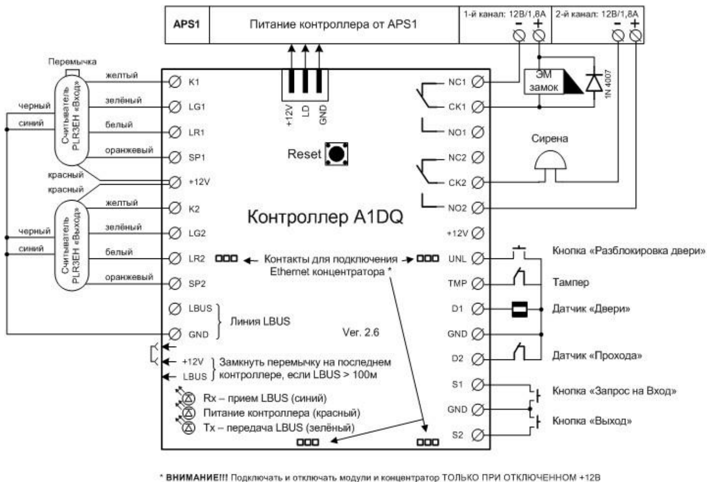
Рисунок 2 – общая схема подключения контроллера A1DQ
