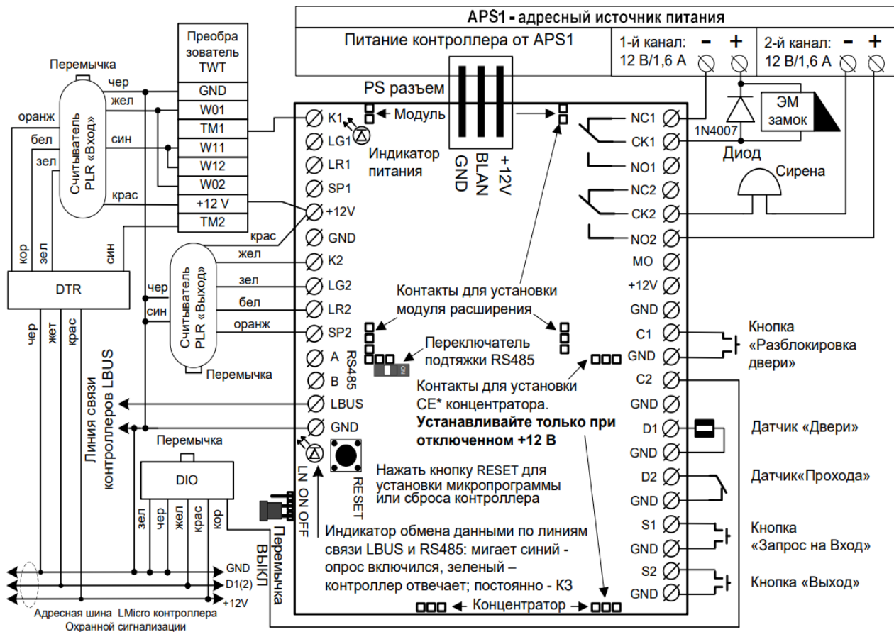
Рисунок 2 – Схема подключения контроллера А1DS/А1DSI
