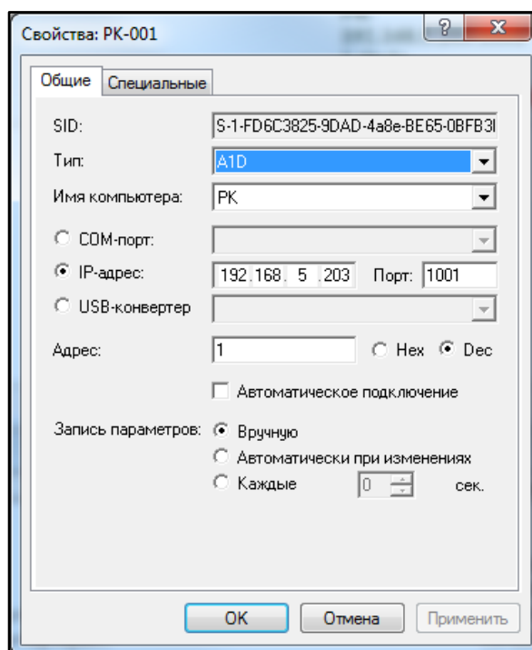
Рисунок 10 – Свойства контроллера
