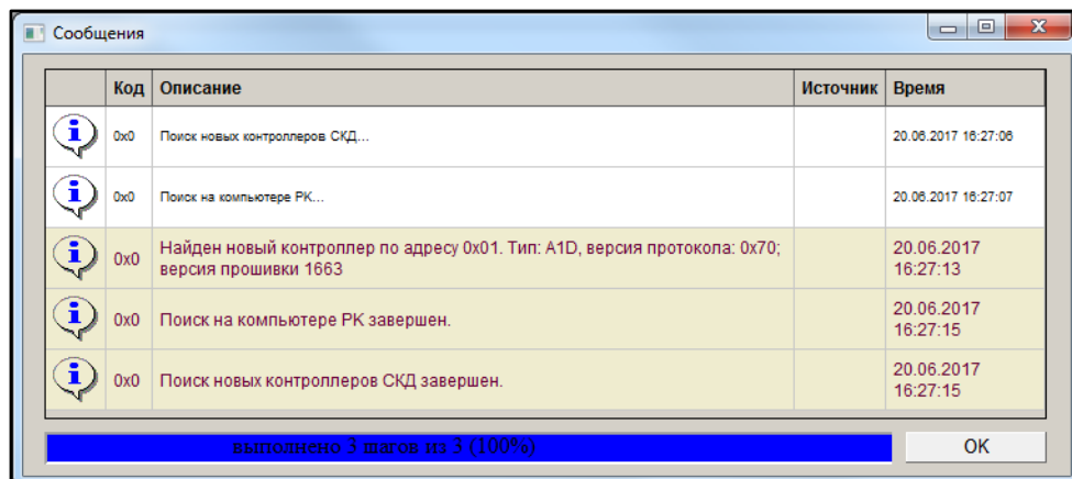
Рисунок 8 – Результаты поиска
