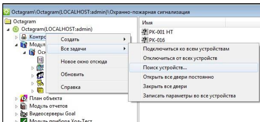
Рисунок 6 – Поиск контроллера.
