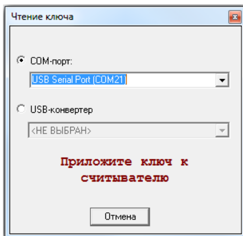
Рисунок 15 – Чтение ключа
