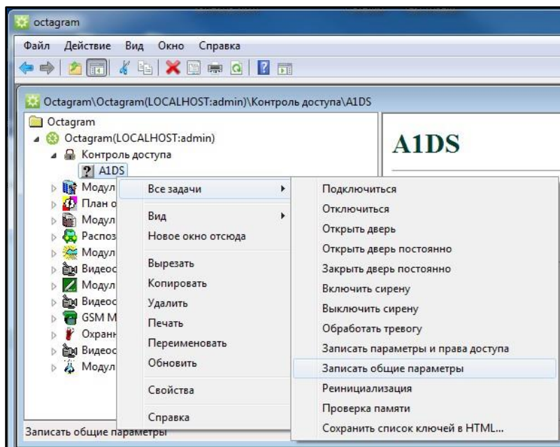
Рисунок 17 – Запись параметров
