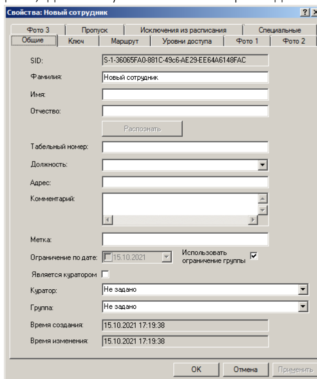
Рисунок 15 – Редактирование сотрудника
