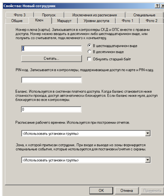
Рисунок 16 – Добавление ключа
