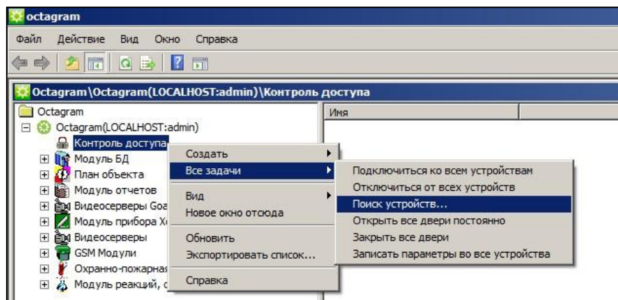
Рисунок 5 – Поиск контроллера.
