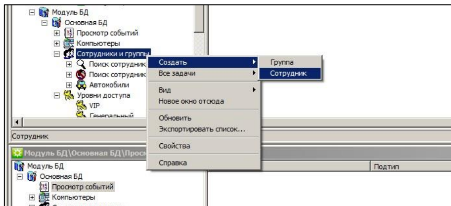
Рисунок 14 – Создание сотрудника
