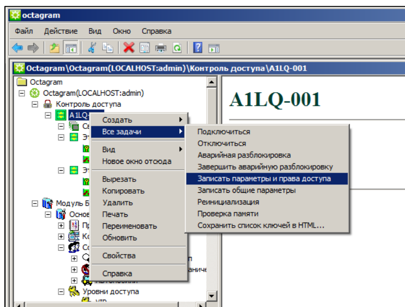
Рисунок 17 – Запись параметров
