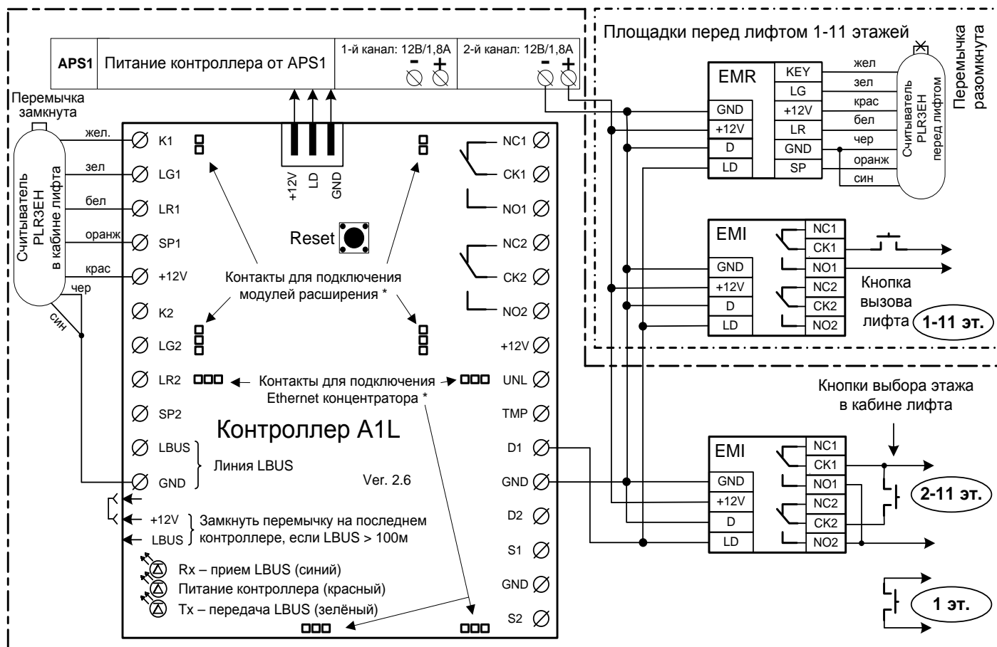
Рисунок 2 Схема подключения.
