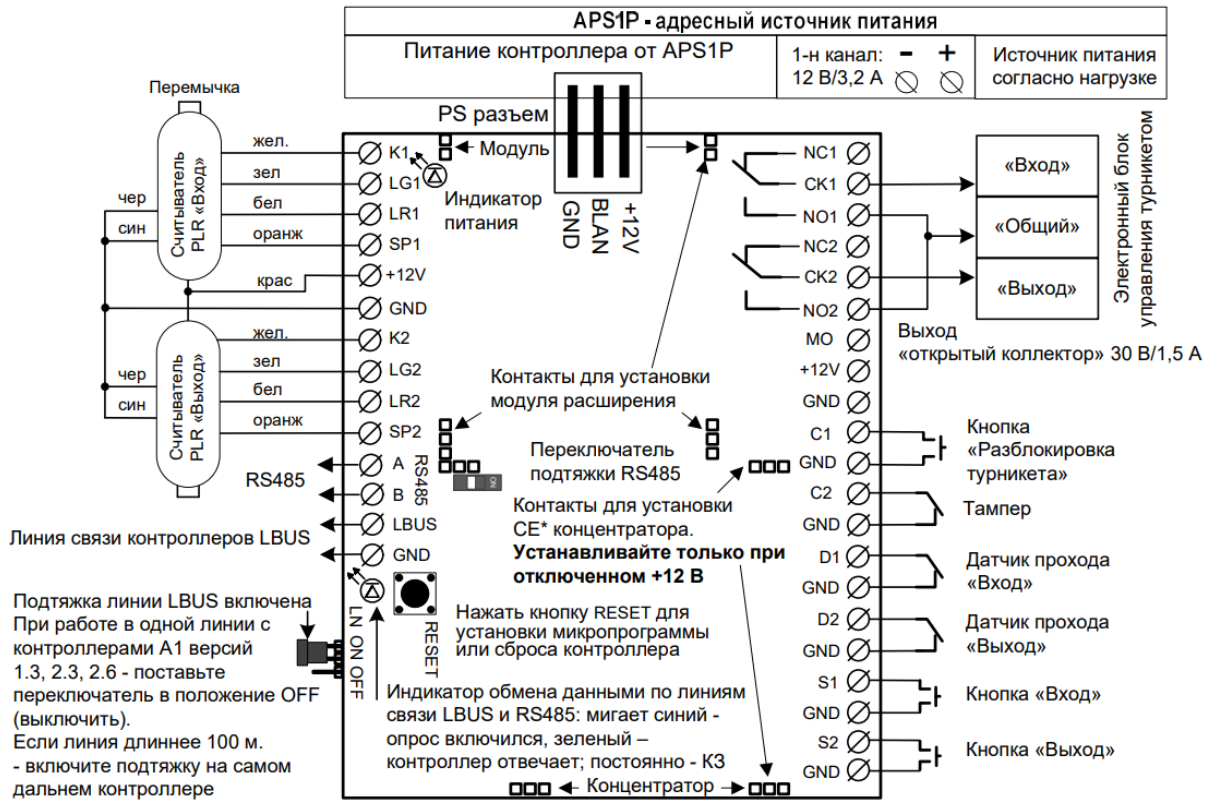
Рисунок 2 – общая схема подключения контроллера А1ТСQ
