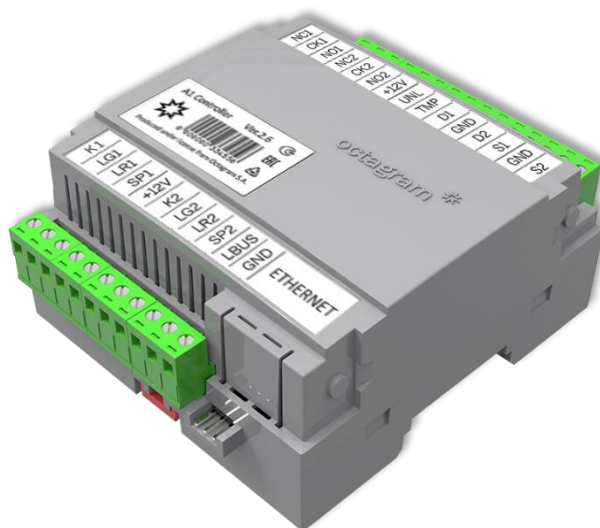
Рисунок 1 – внешний вид контроллера A1TCQ без модуля 4S2R.
