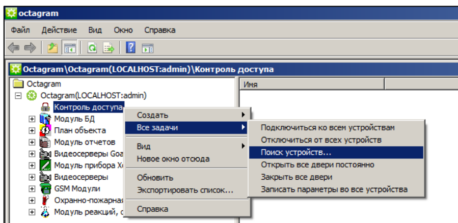
Рисунок 5 – Поиск контроллера.
