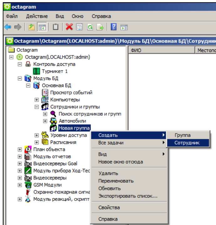
Рисунок 21 – Создание сотрудника
