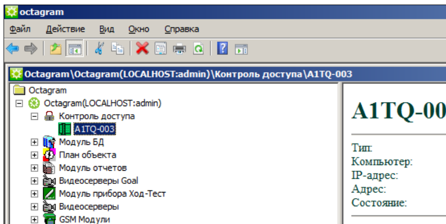
Рисунок 7 – Контроллер добавлен
