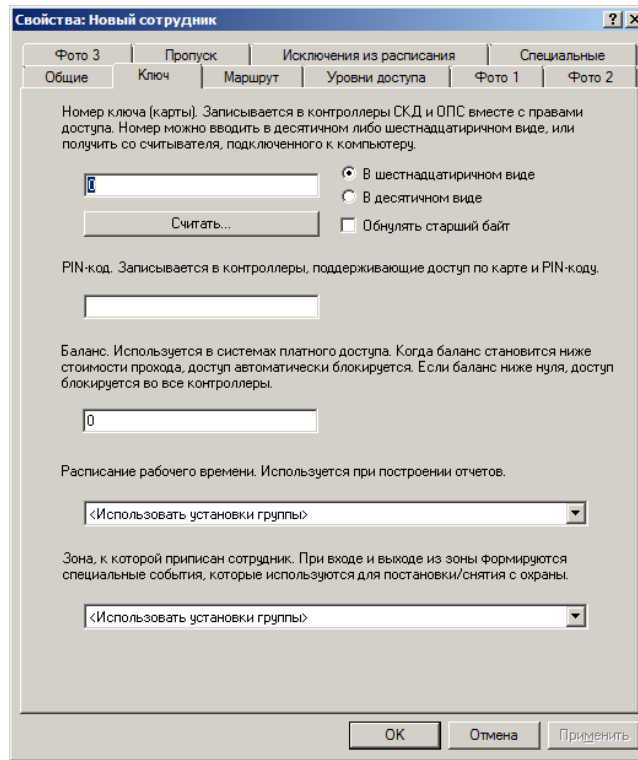
Рисунок 23 – Добавление ключа
