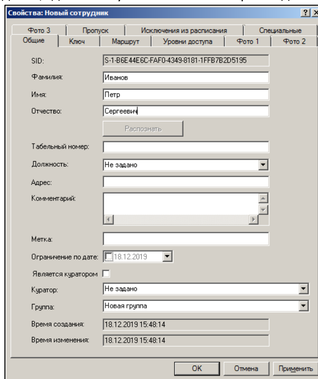
Рисунок 22 – Редактирование сотрудника
