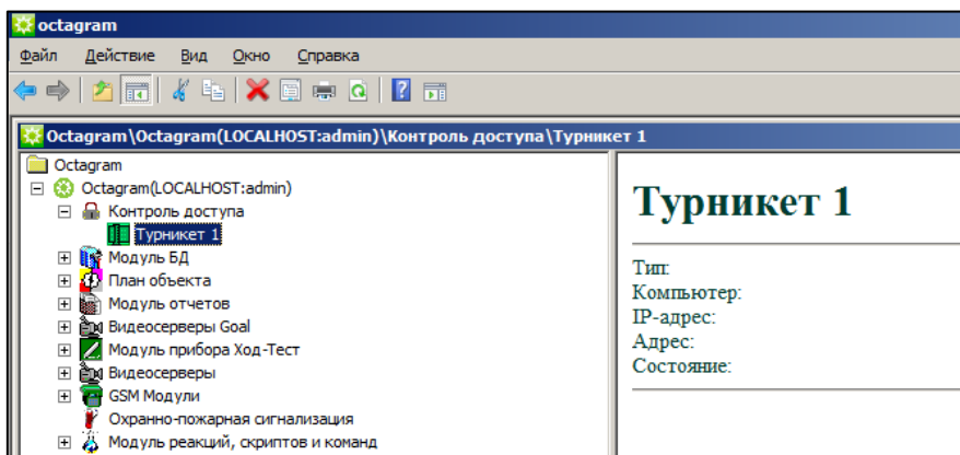
Рисунок 8 – Переименованный контроллер
