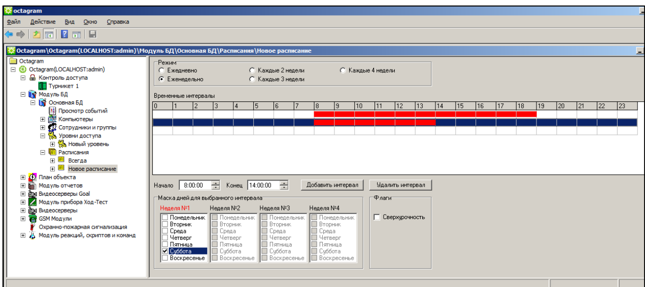
Рисунок 17 – Настройка расписания
