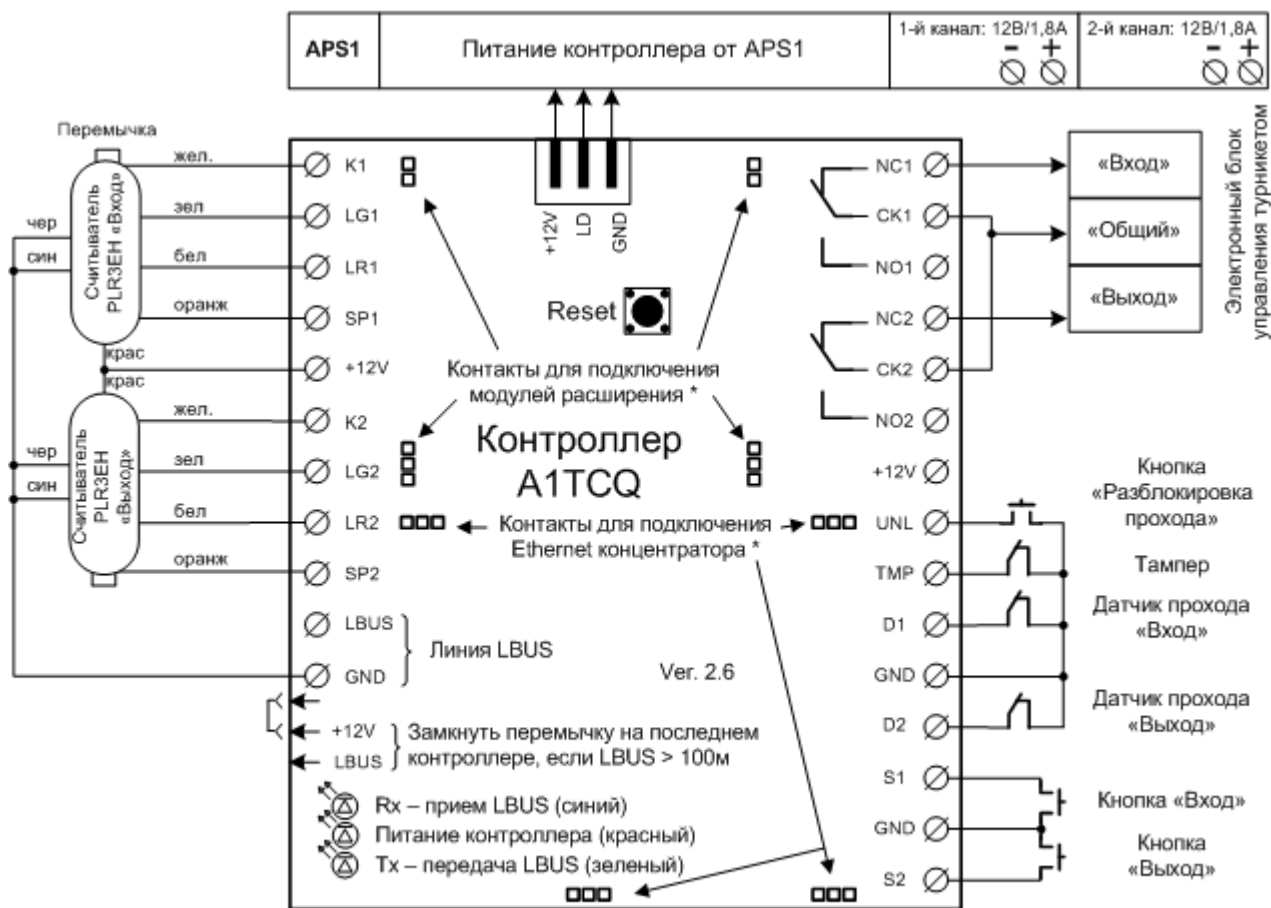
Рисунок 2 – общая схема подключения контроллера А1ТСQ
