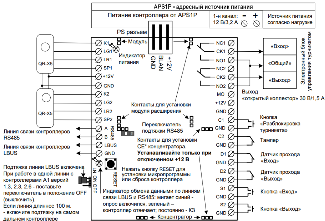
Рисунок 2 – Схема подключения контроллера A1TX
