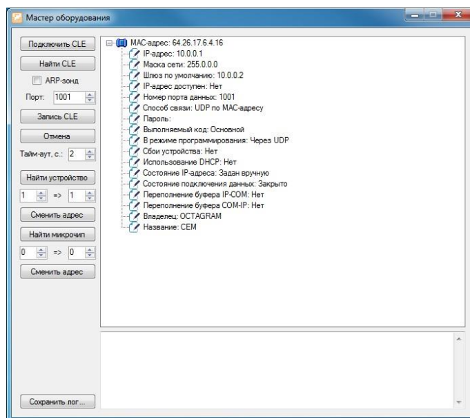
Рисунок 7 - Настройка концентратора
