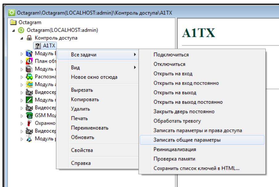
Рисунок 14 – Запись параметров
