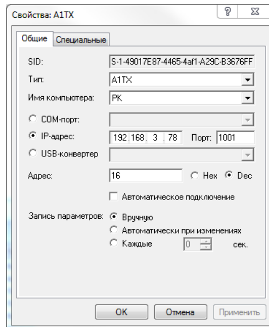
Рисунок 12 – Свойства контроллера
