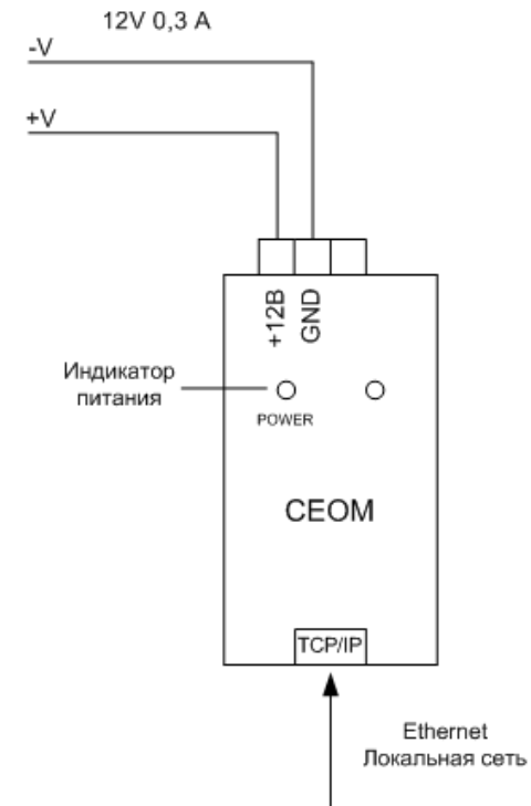
Рисунок 1 Схема подключения CEOM
