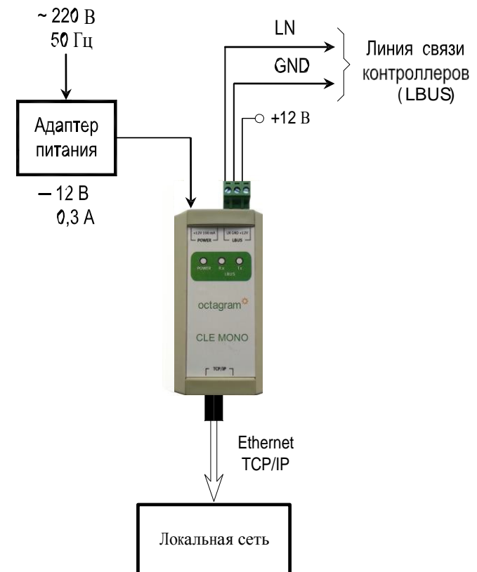
Рис. 1. Схема подключения конвертера CLEMP
