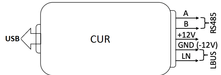
Рис.1. Схема подключения конвертера CUR
