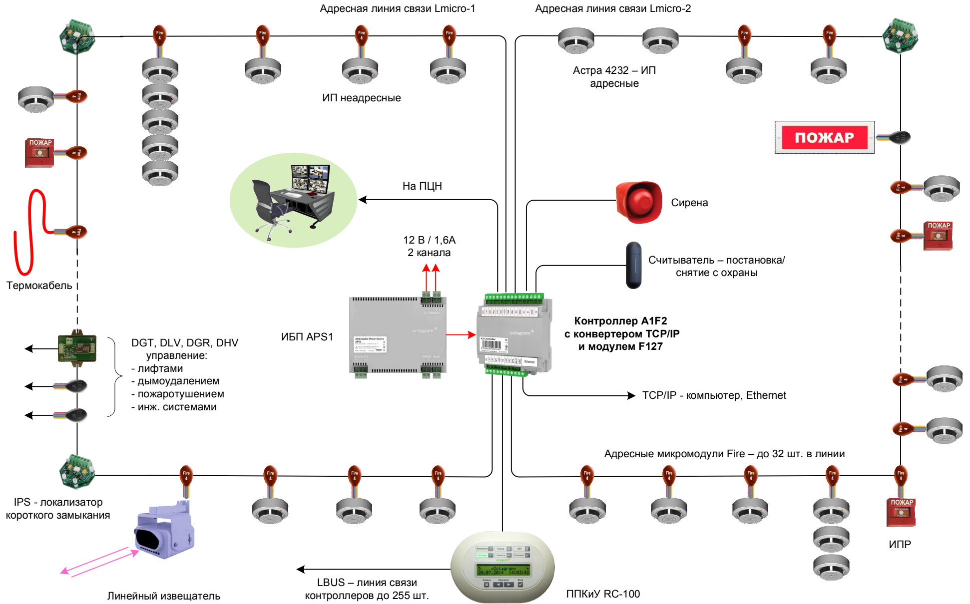
Система автоматической пожарной сигнализации на контроллере A1F2
