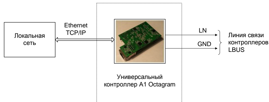
Рис. 1. Схема подключения платы IP концентратора - конвертера CED
