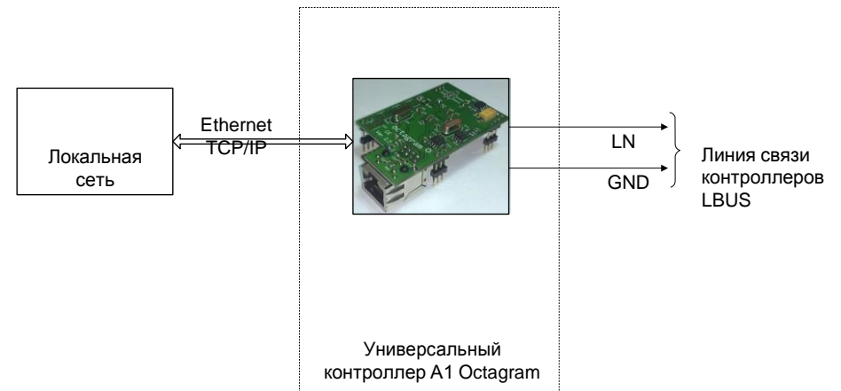
Рис. 1. Схема подключения платы IP концентратора - конвертера СЕМР
