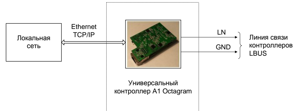
Рис. 1. Схема подключения платы IP концентратора - конвертера СЕМ
