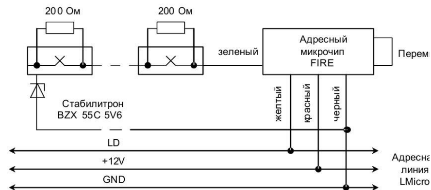
Рис.3. Схема подключения пожарных тепловых извещателей с нормально замкнутыми контактами
