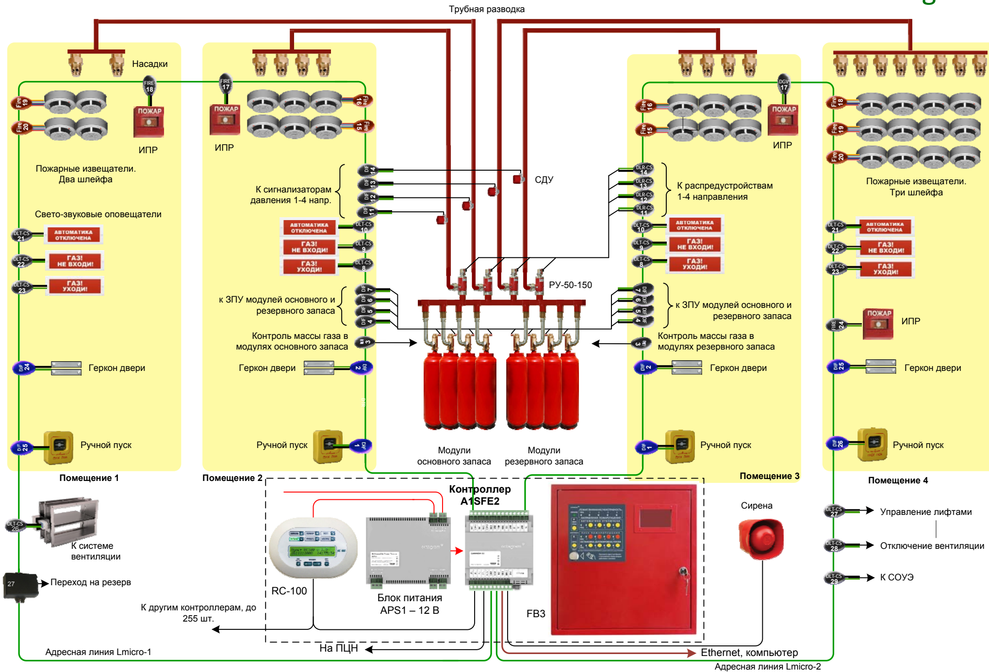
Автоматическая система газового пожаротушения (АУГП) на 4 направления
