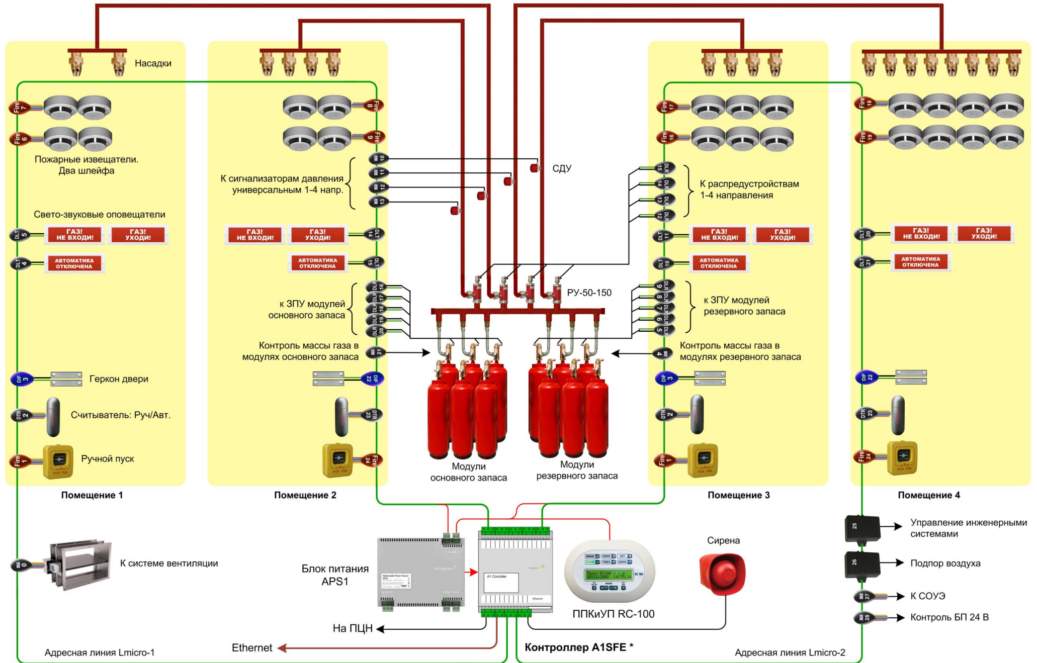
Автоматическая система газового пожаротушения (АУГП) на 4 направления
