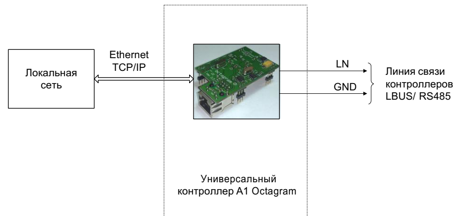
Рис. 1. Схема подключения платы IP концентратора - конвертера CE
