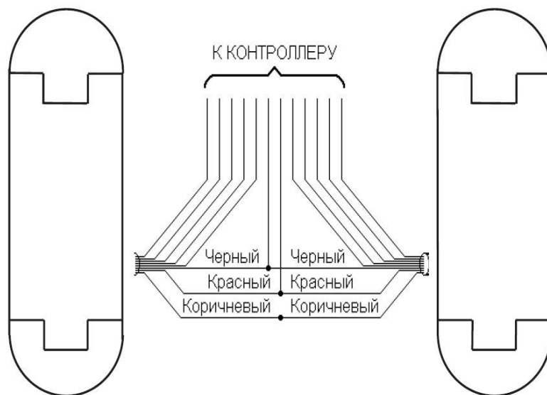
Схема подключения
